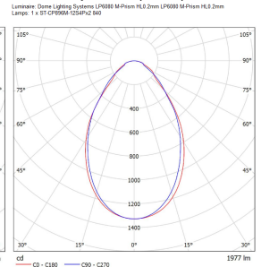
MP—2 Layer Prism (UGR19)/1m, 18.4W
